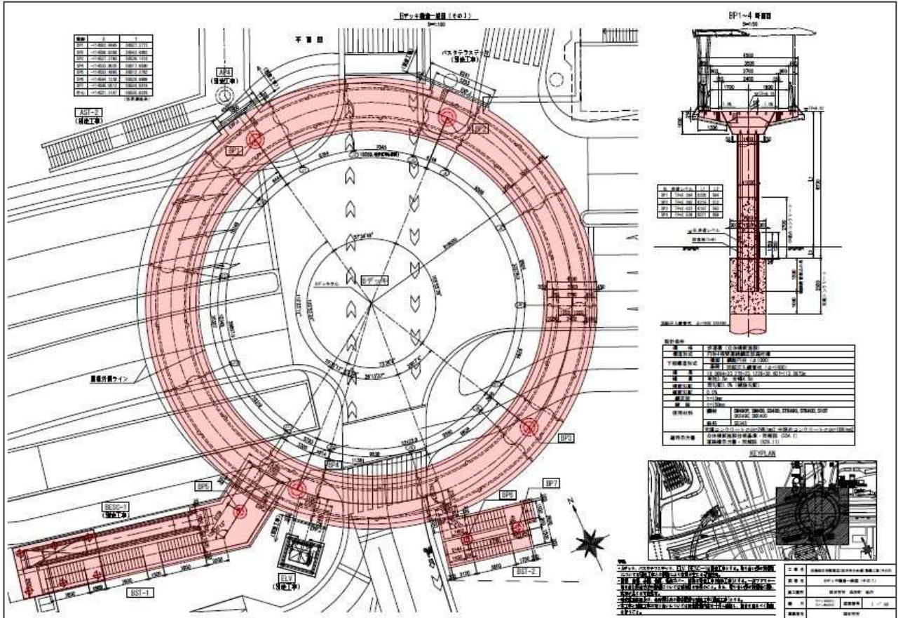
近鉄四日市駅周辺（四日市中央線）整備工事（その5）
