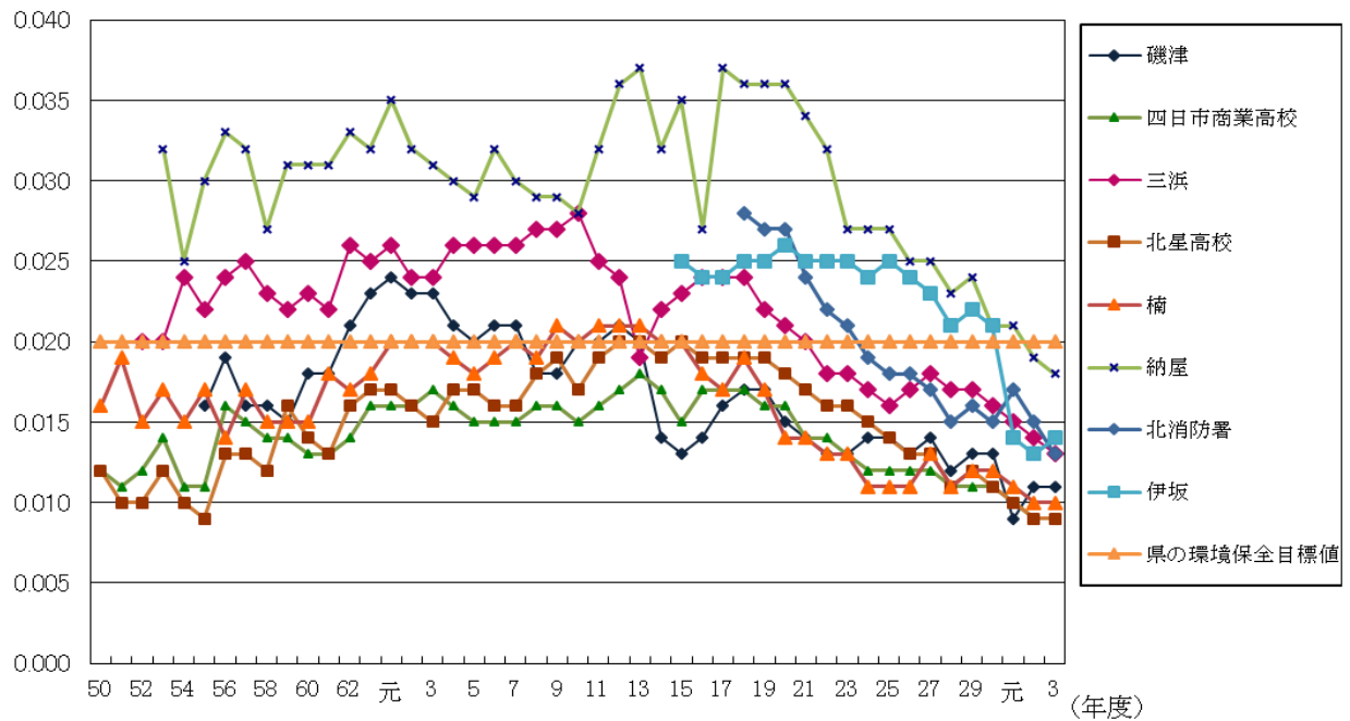
二酸化窒素濃度(年平均値)の経年変化
