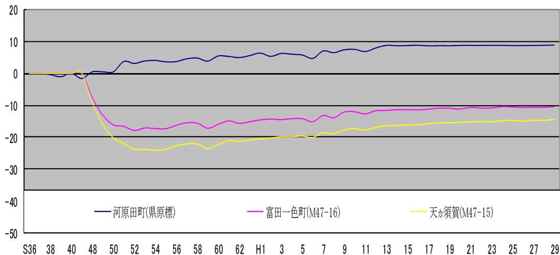
ア 地盤沈下量(累積変動量:cm)
