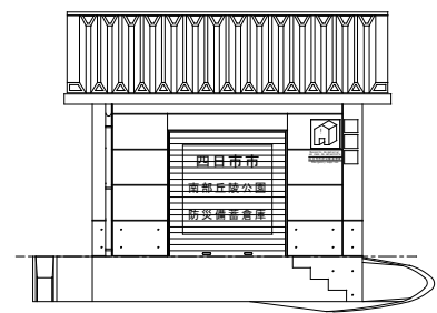
南西立面図
