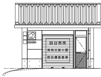
北東立面図
